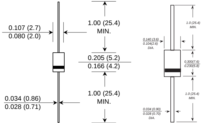
CASE DO-41
